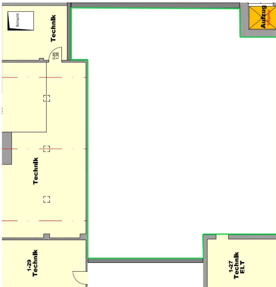
Grundriss Lagerhalle (grün markiert)
