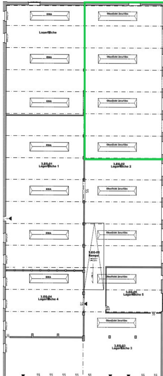
Grundriss Teilfläche einer Lagerhalle mit 6 Rampen (grün markiert)
